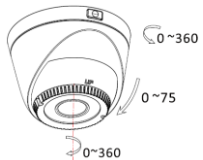
Рисунок 1-21 Настройка угла наблюдения камеры
