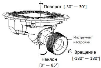
Рисунок 1-23 Настройка угла наблюдения камеры
