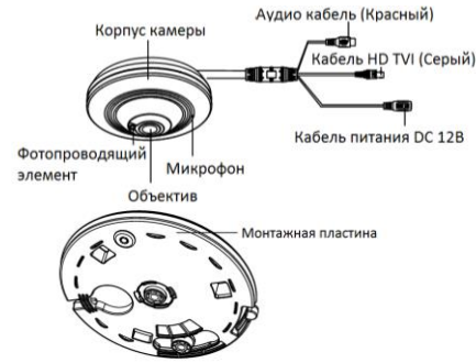
Рисунок 1-26 Панорамная камера
